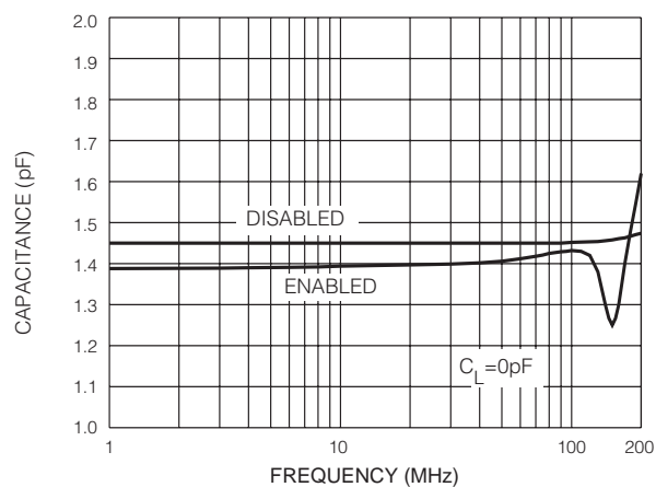
Fig. 3 Input Capacitance
