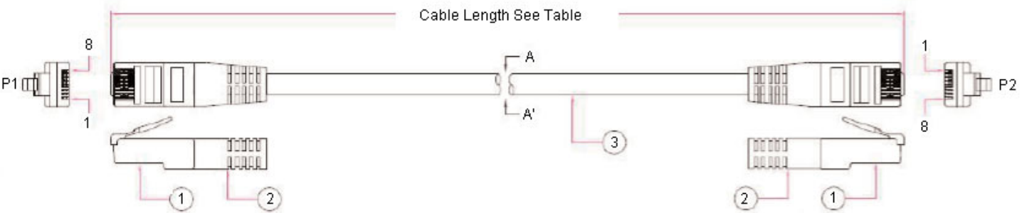
Wiring
