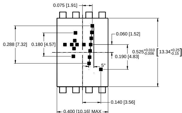
4N53
