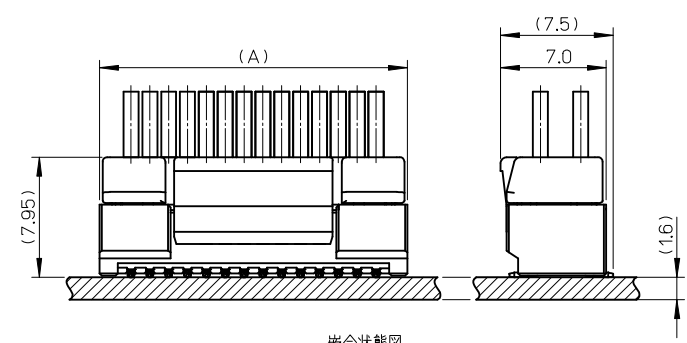
嵌合状態図 MATED CONNECTORS
