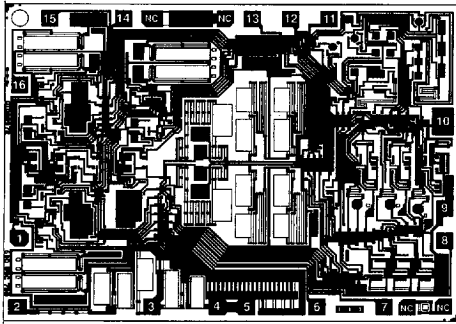
INA102 DIE TOPOGRAPHY
