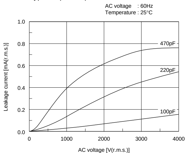
Type KJ (B char.)
