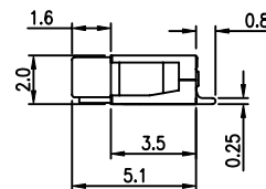
ACTUATOR CLOSE
