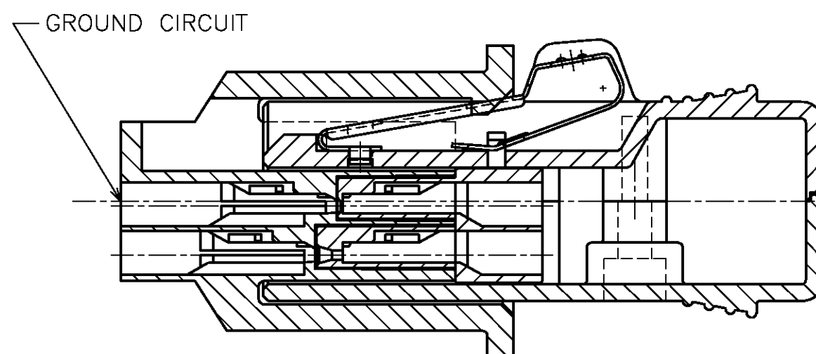
B-B (SCALE 2:1)
