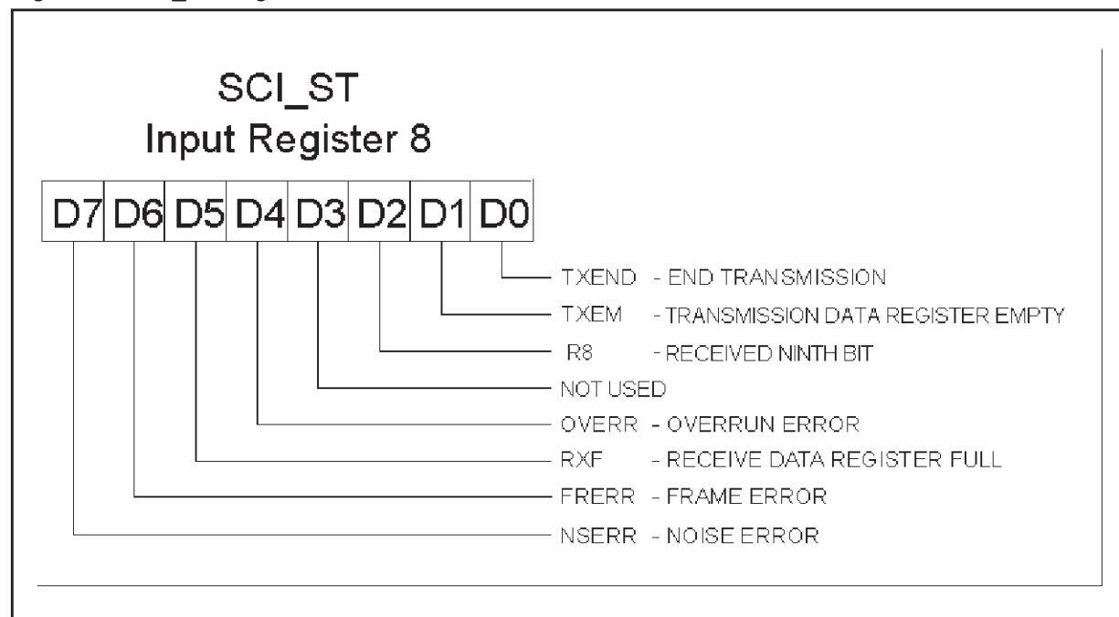
Figure 2.7. SCI_ST Registers
