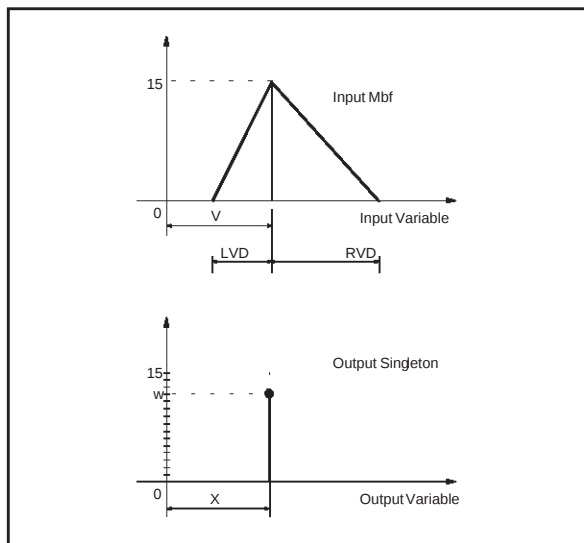
Figure 2.12. Mbfs Parameters
