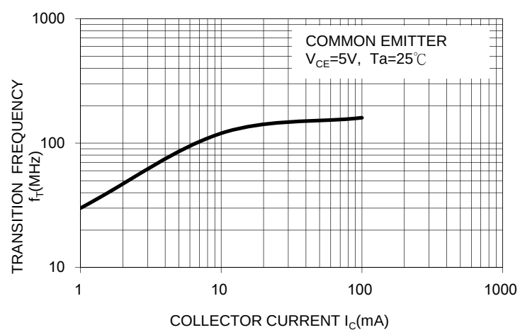
FIG.8 f_T - I_C
