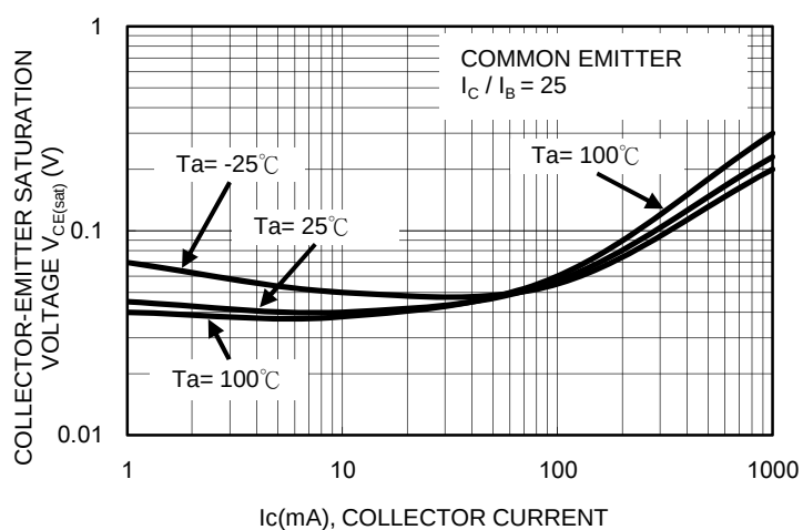
FIG. 6 V_{CE(sat)} - I_C
