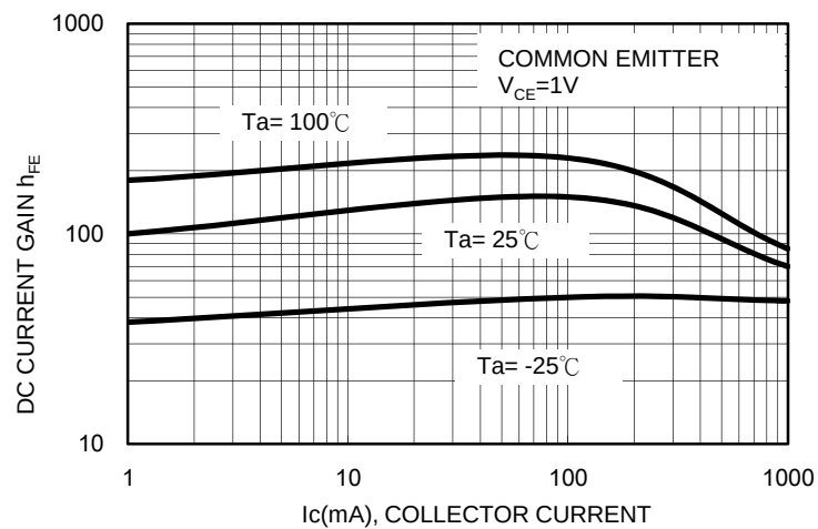
FIG. 4 h_{FE} - I_C
