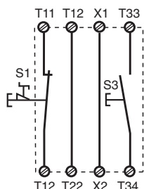
Fig. 2: Circuito de entrada monocal/Circuito di entrata monocalale/Eenkanalig ingangscircuit
