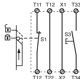
Fig. 4: Control puerta protectora monocal/ Controllo porta di sicurezza monocalale/ Eenkanalige hekbewaking
