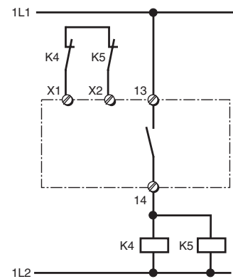
Fig. 9: Anschlußbeispiel für externe Schütze/ Connection example for external contactors, relays/Branchement contacteurs externes
