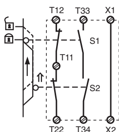
Fig. 6: Control puerta de protección, rearme automático/Controllo porta di sicurezza bicanale, start automatico/Tweekanalige hekbewaking, automatische start
