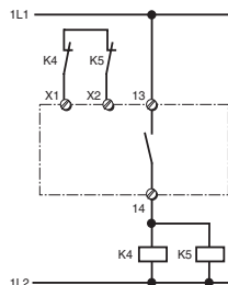
Fig. 3: Circuito de entrada bicanal/Circuito d'ingresso bicanale/Tweekanalig ingangscircuit
