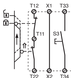
Fig. 5: Control de puerta protectora bicanal/ Comando porta di sicurezza bicanale/ Tweekanalige hekbewaking
