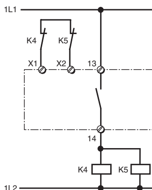
Fig. 9: Ejemplo de conexión para contactores externos/Esempio di collegamento per relè esterni/Aansluitvoorbeeld voor externe magneetschakelaars
