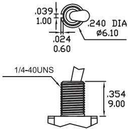
B7 LONG
