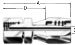
Metric universal female swivel 24° DIN 3901/3902 s.Rh. 07.155-
