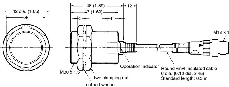
Fig. 24: E2E-X20MD1-M1GJ-N
