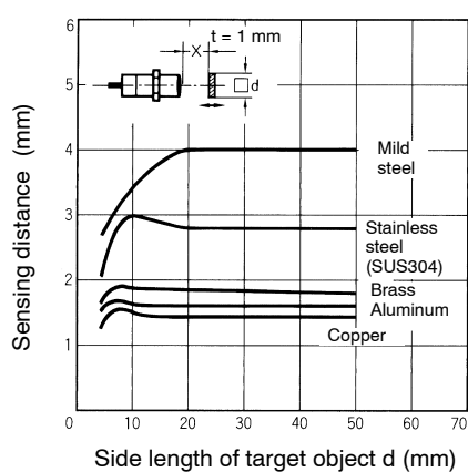
E2E-X4MD□-N
