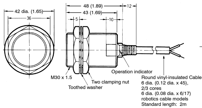
Fig. 7: E2E-X10D□-N
