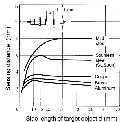
E2E-X8MD□-N
