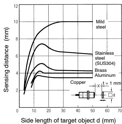
E2E-X10D□-N
