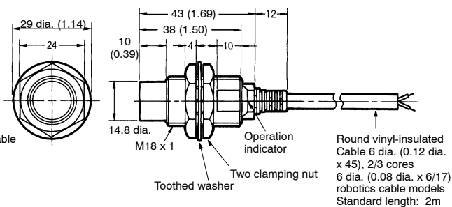
Fig. 6: E2E-X14MD□
