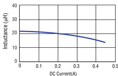
SRN2010TA-220M
