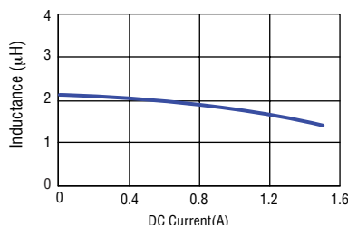
SRN2010TA-2R2M
