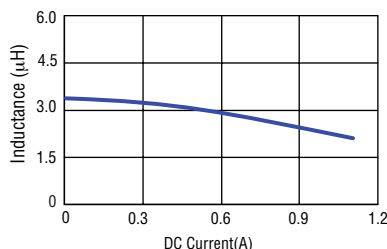
SRN2010TA-3R3M
