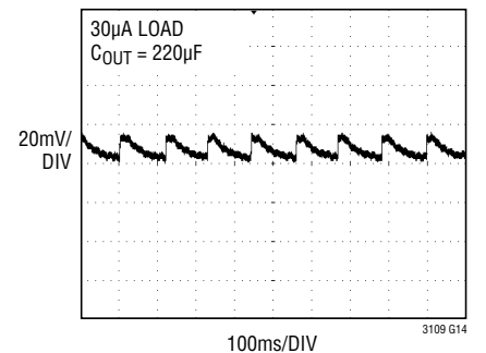
V_{OUT} Ripple
