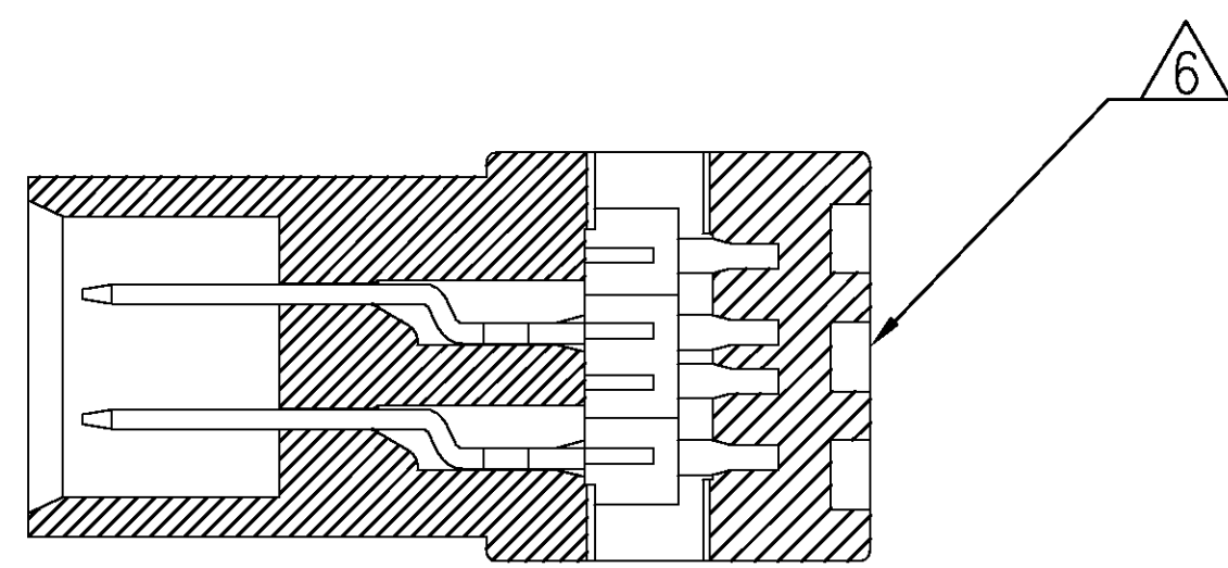
SEC. A-A
