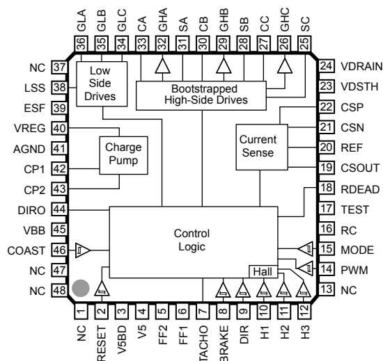
JP Package
