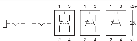
Wiring diagram 277
