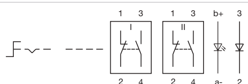
Wiring diagram 279
