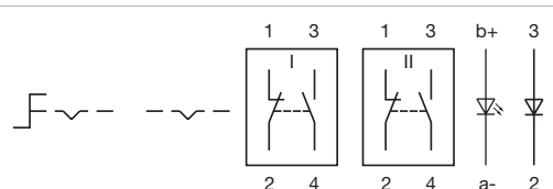
Wiring diagram 281
