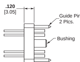
Receptacle
