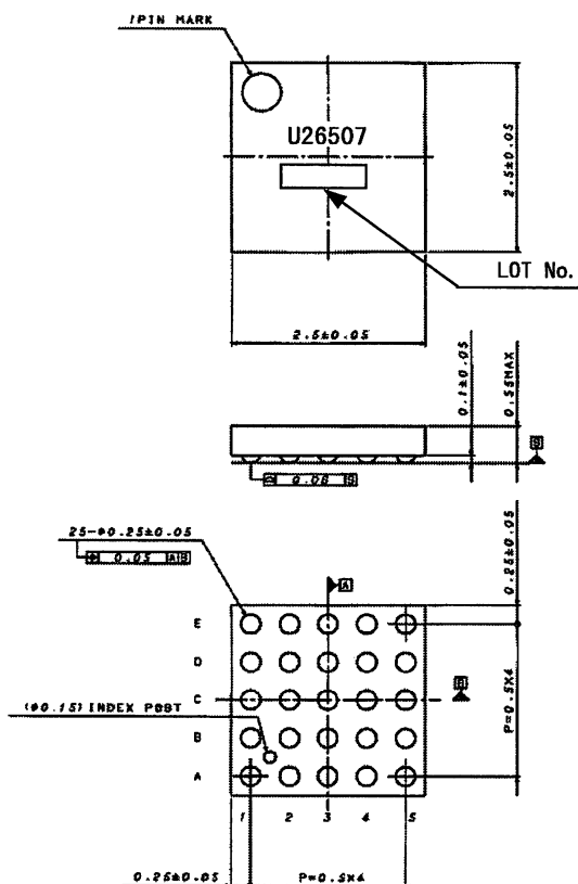
VCSP50L2 ( Unit:mm )
