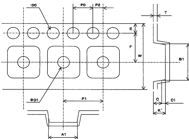
Fig. 3 Tape dimensions
