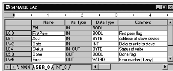
Bild 6-38 Lokale Variablentabelle
