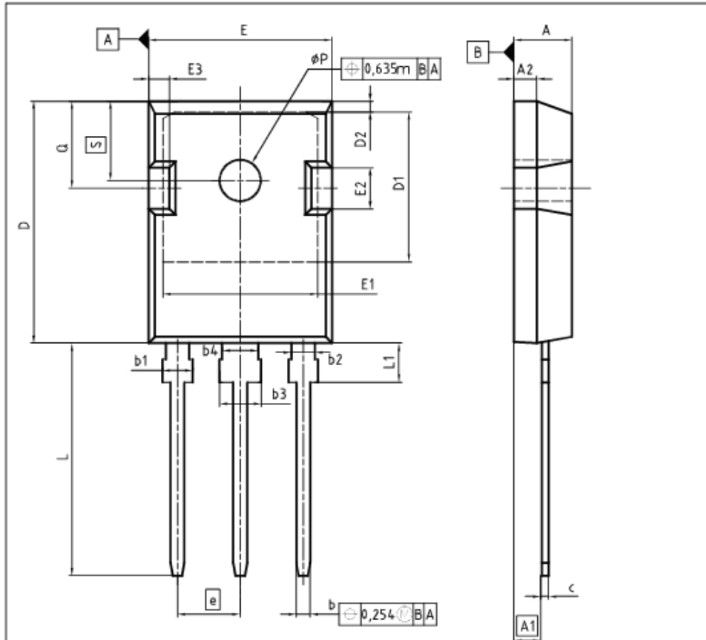
TO247-3
