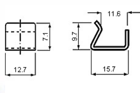
FIG. Metal Clip
