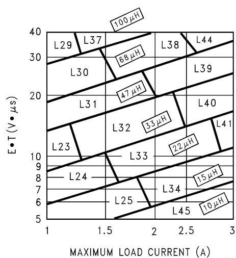
Figure 24. LM2670-ADJ
