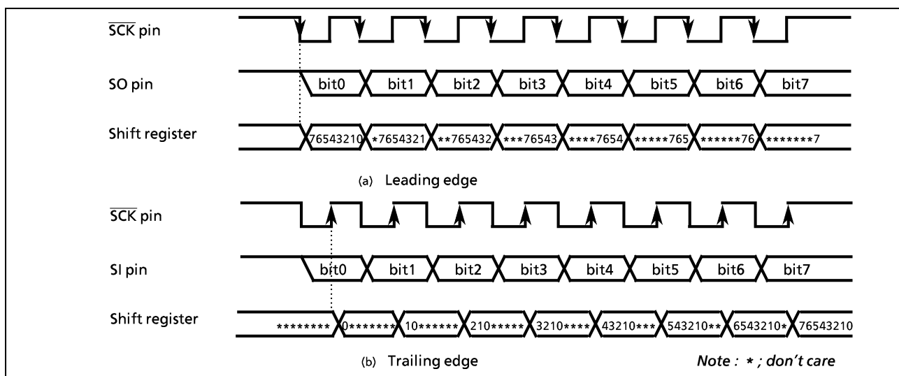
Figure 2-46. Shift edge
