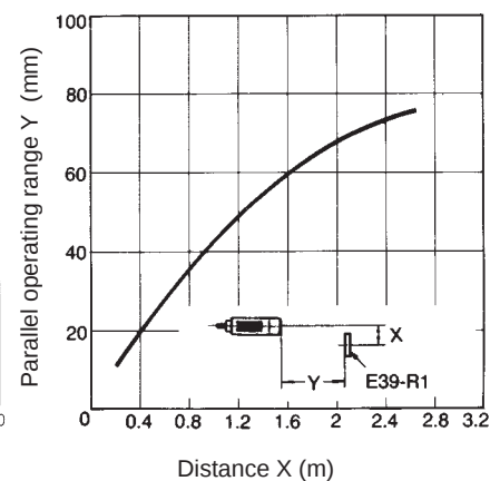
E3S-R2E4(1)
