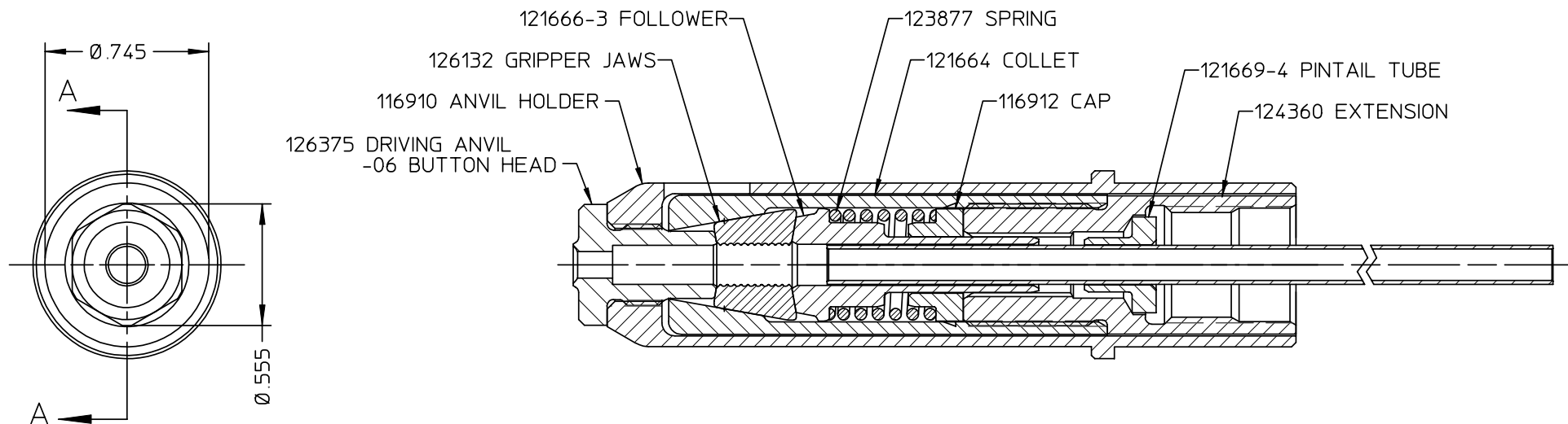
SECTION A-A
