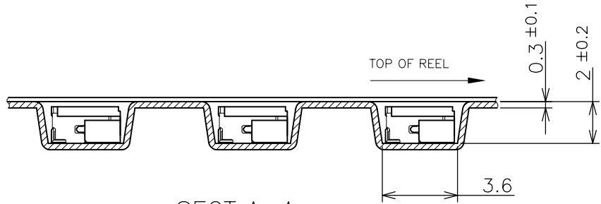
SECT A-A (SCALE 4:1)
