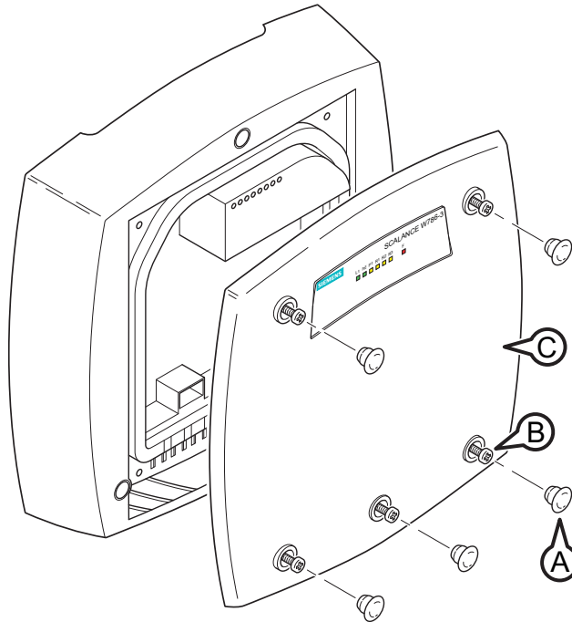
Bild 3-1 Deckeldemontage A Verschlusskappe B Deckelverschraubung C Gehäusedeckel
