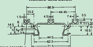
Bezel Section
