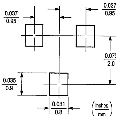
SOT-23
