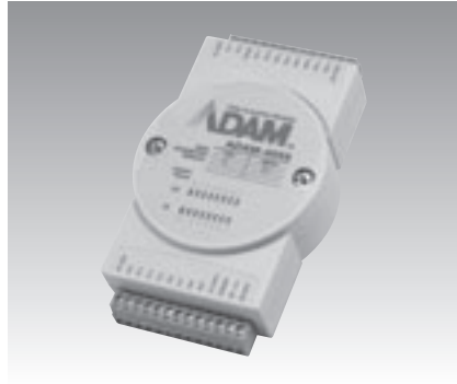
ADAM-4055
