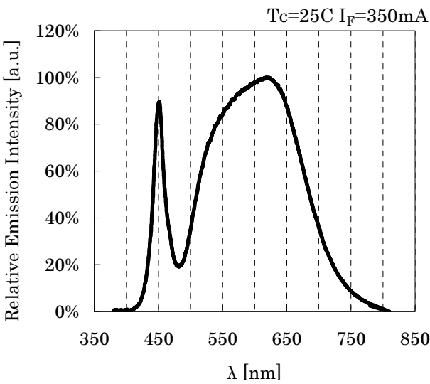
•Spectrum
