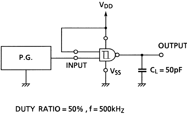
測定回路
