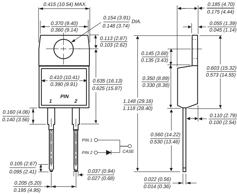
TO-220AC (UG8AT-DT)
