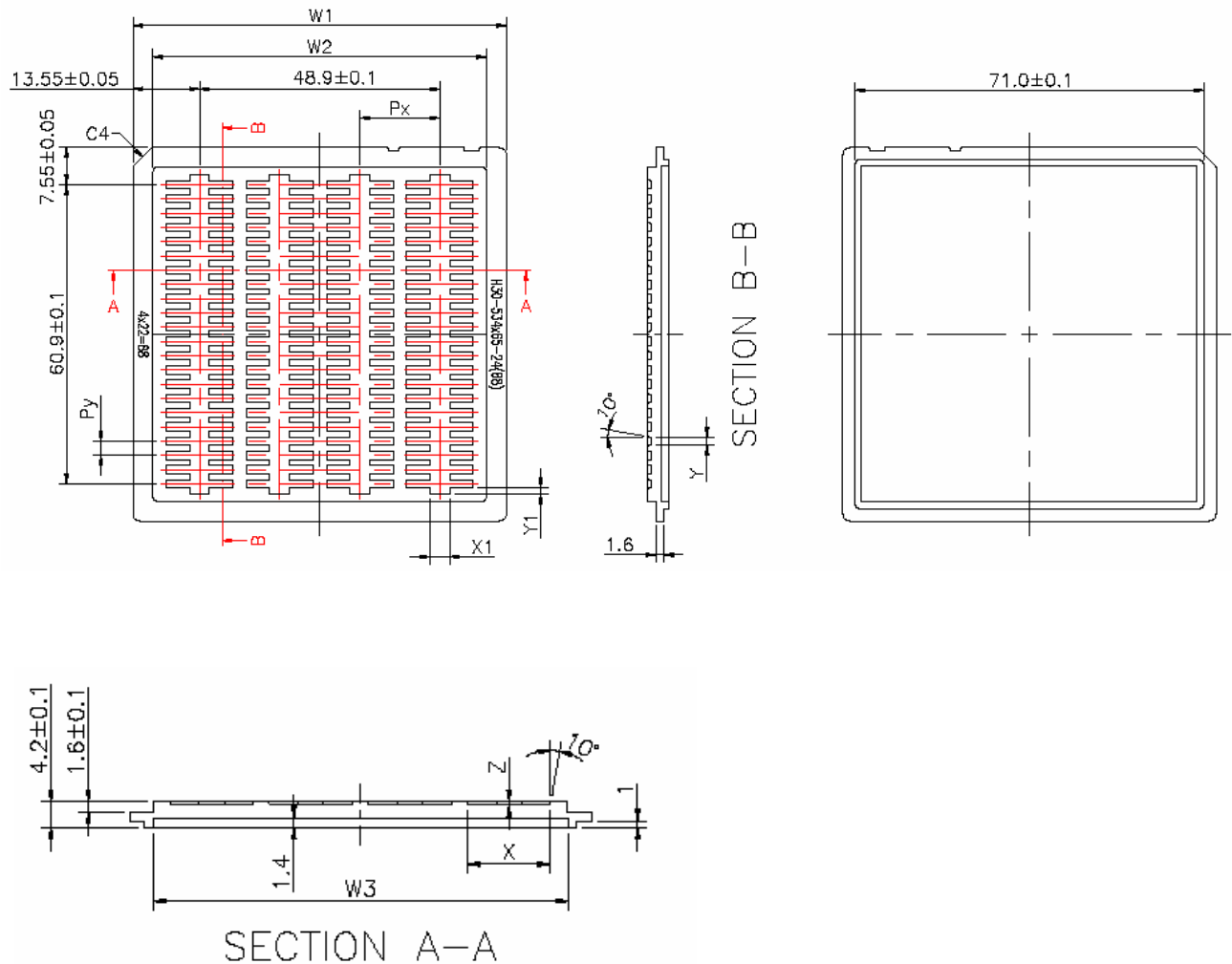
Figure 15-1 : Die Tray Information
