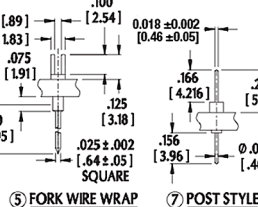
⑤ FORK WIRE WRAP
