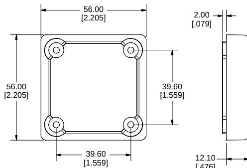
BOTTOM OF LID
