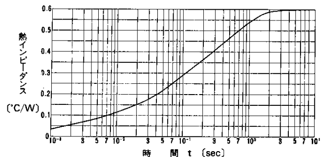
過渡熱インピーダンス (接合—ケース間)
