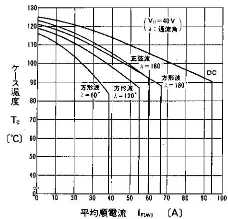
平均順電流—ケース温度 (50Hz)
