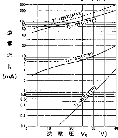
逆特性
