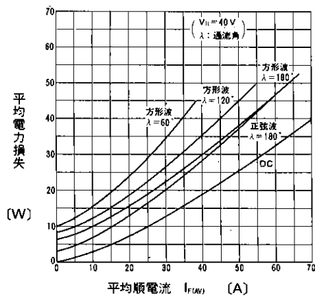
平均電力損失
