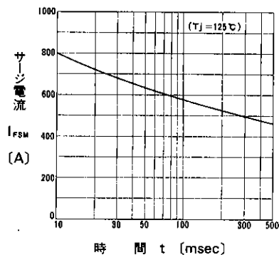
サージ電流 (50Hz 正弦波)
