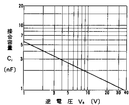
接合容量
