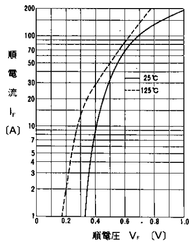
順特性
