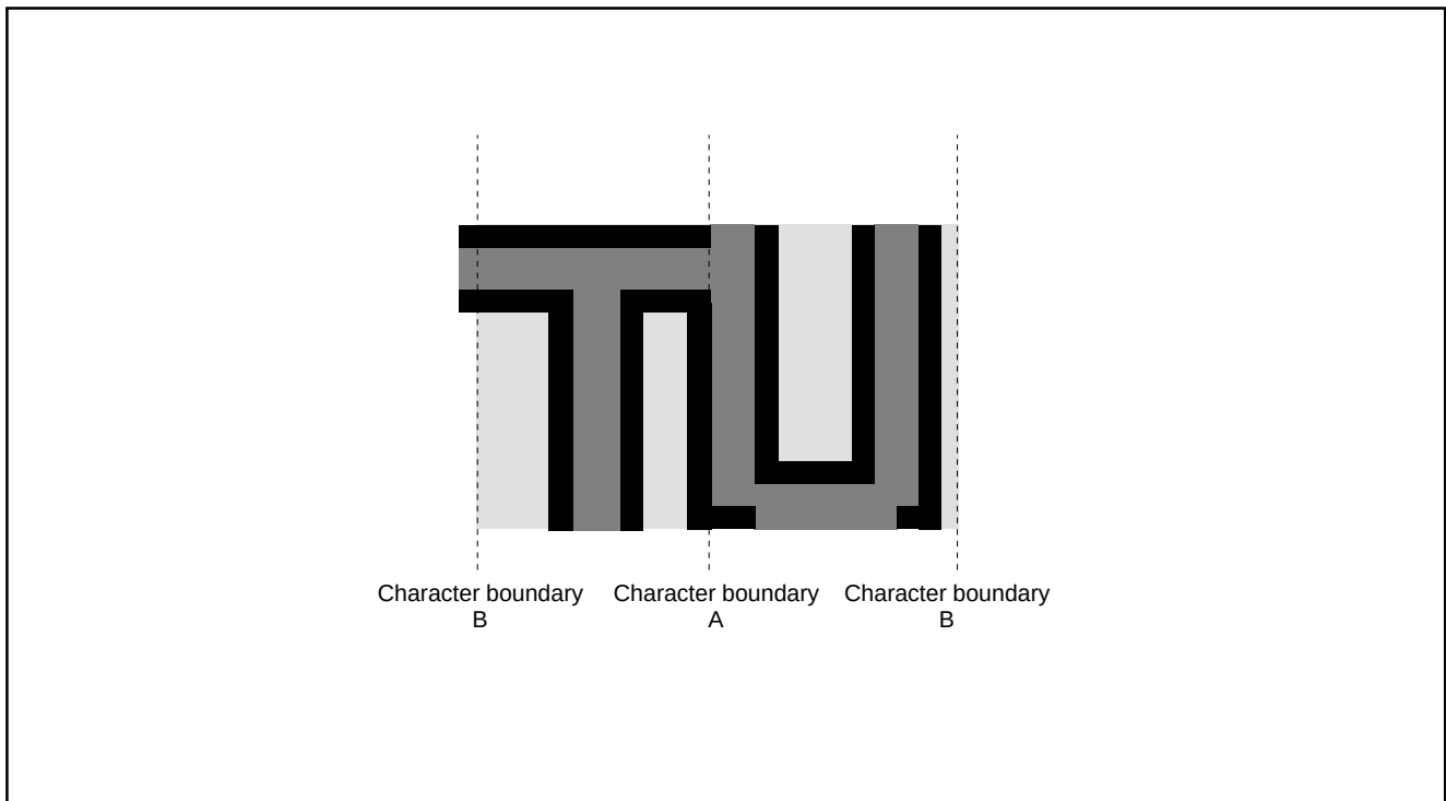
Fig. 8.11.23 Border Priority
