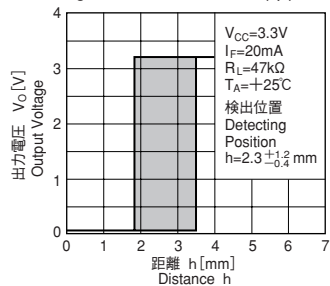
検出位置特性 (1) (参考)
