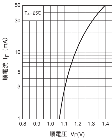
順電流—順電圧特性 (標準値)
