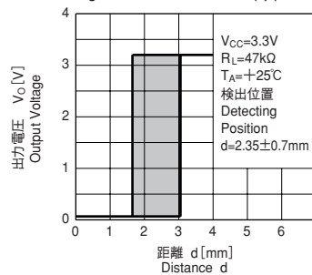
検出位置特性 (2) (参考)
