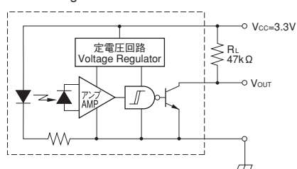
※応答時間測定回路
