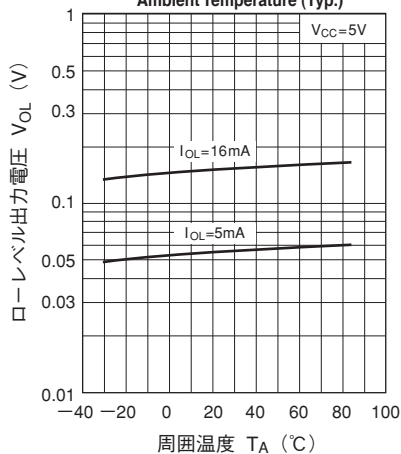
ローレベル出力電圧—周囲温度特性 (標準値) Low Level Output Voltage vs. T_A Ambient Temperature (Typ.)
