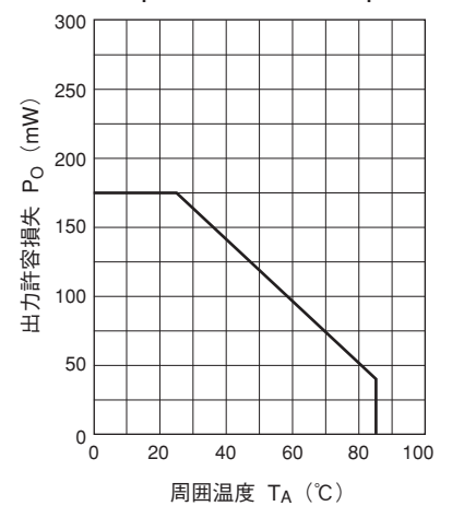
出力許容損失低減曲線
