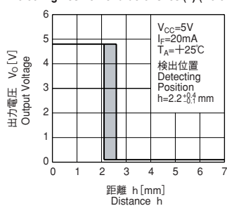
検出位置特性 (1) (参考)
