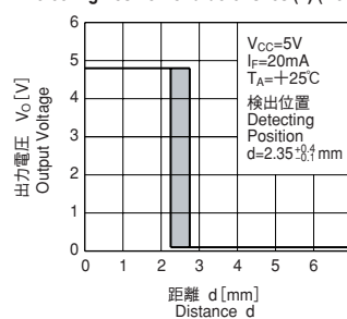
検出位置特性 (2) (参考)
