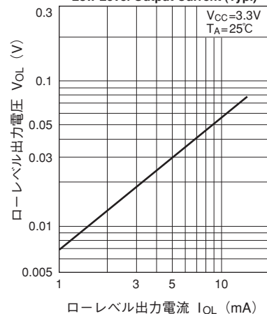
ローレベル出力電圧—ローレベル出力電流特性 (標準値) Low Level Output Voltage vs. I_{OL} Low Level Output Current (Typ.)
