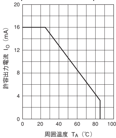
出力電流低減曲線
