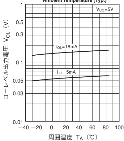
ローレベル出力電圧—周囲温度特性 (標準値) Low Level Output Voltage vs. \square Ambient Temperature (Typ.)
