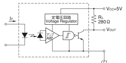
※2 応答時間測定回路
