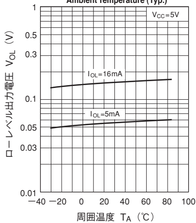
ローレベル出力電圧—周囲温度特性 (標準値) Low Level Output Voltage vs. T_A Ambient Temperature (Typ.)
