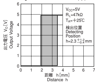
検出位置特性 (1) (参考)
