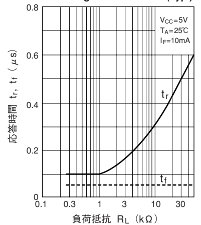
応答時間—負荷抵抗特性 (標準値)
