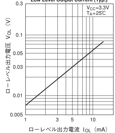
ローレベル出力電圧—ローレベル出力電流特性 (標準値)
