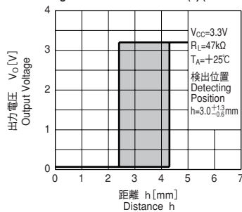
検出位置特性 (1) (参考)
