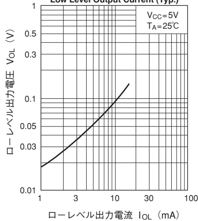
ローレベル出力電圧—ローレベル出力電流特性 (標準値) Low Level Output Voltage vs. \square Low Level Output Current (Typ.)
