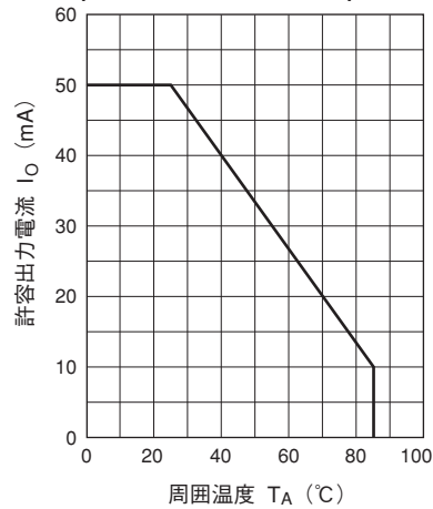
出力電流低減曲線
