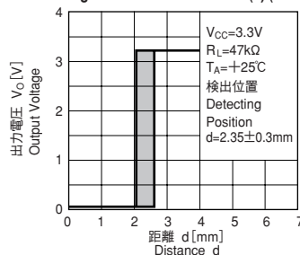
検出位置特性 (2) (参考)
