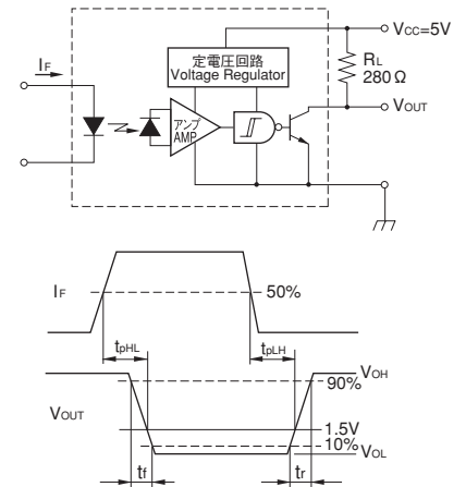
※2 応答時間測定回路
