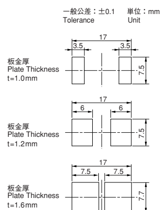
取り付け穴寸法 (参考)
