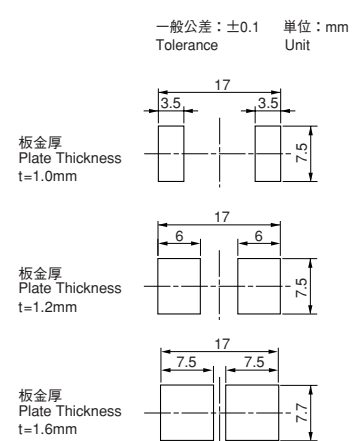
取り付け寸法 (参考)
