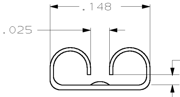
SECT A-A
