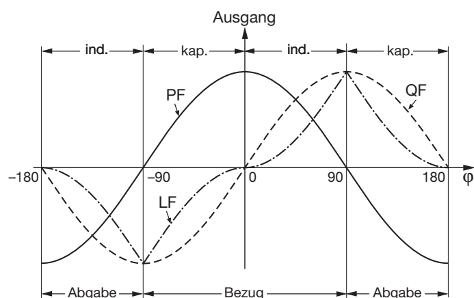
Bild 7. Wirkfaktor PF —, Blindfaktor QF -----, Leistungsfaktor LF -----.
