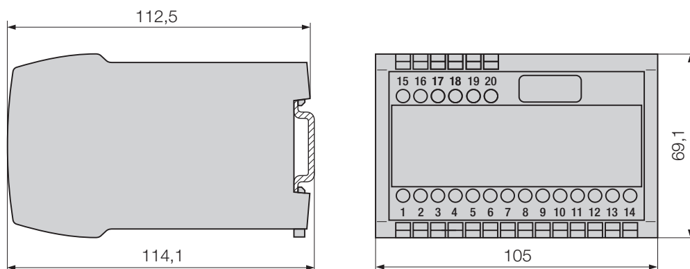
Bild 6. SINEAX M 563 im Gehäuse P20/105 auf Hutschiene (35 \times 15 mm oder 35 \times 7,5 mm, nach EN 50 022) aufgeschnappt.
