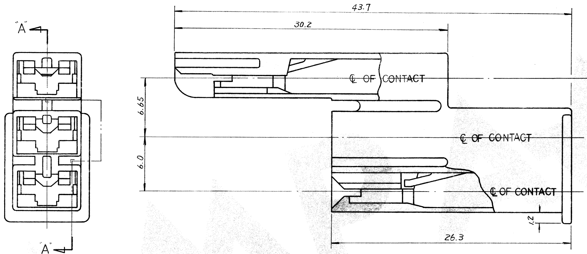
断面 "A-A"
