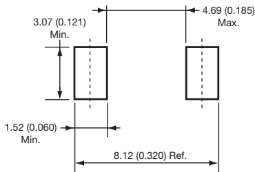
DO-214AB (SMC)
