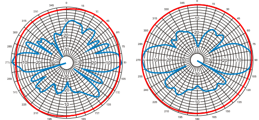
5.5 GHz H-Plane E-Plane 2.45 GHz
