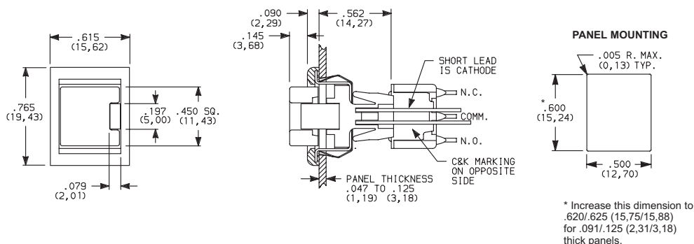
8161J86ZQE223 SPDT
