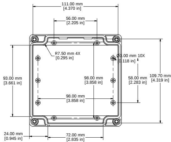
LID - INSIDE
