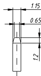
Detail Y
